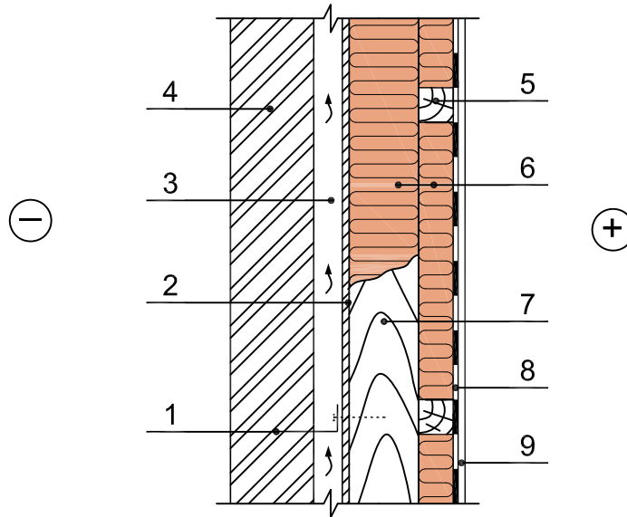
Vertikalus pjūvis
