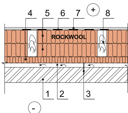
Horizontalus pjūvis
