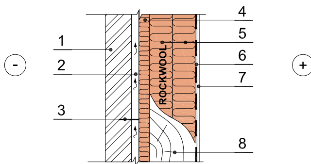
Horizontalus pjūvis
