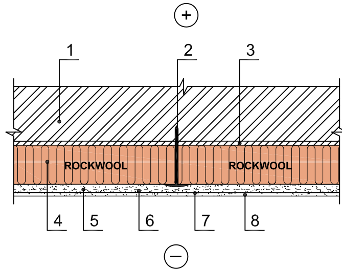
Horizontalus pjūvis
