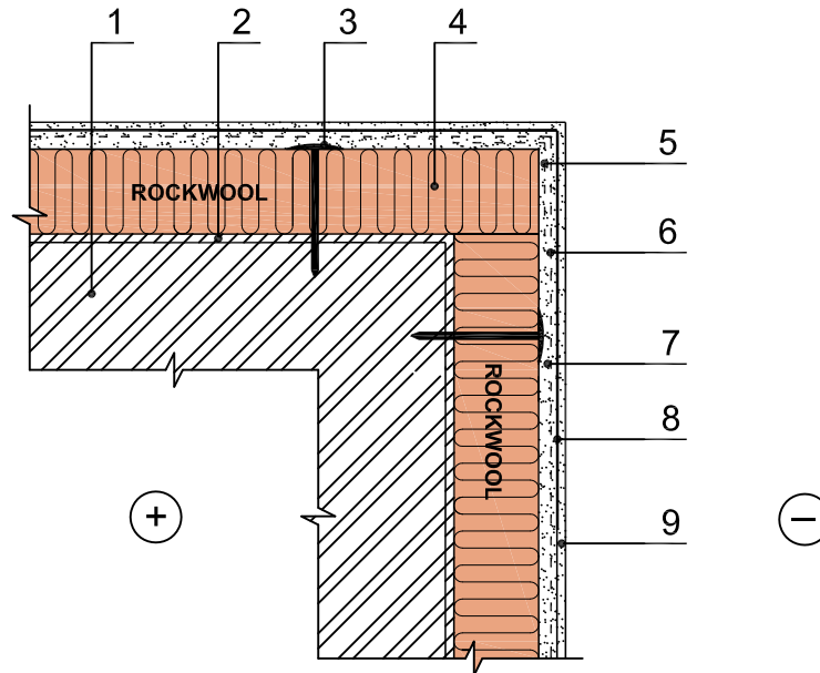
Horizontalus pjūvis
