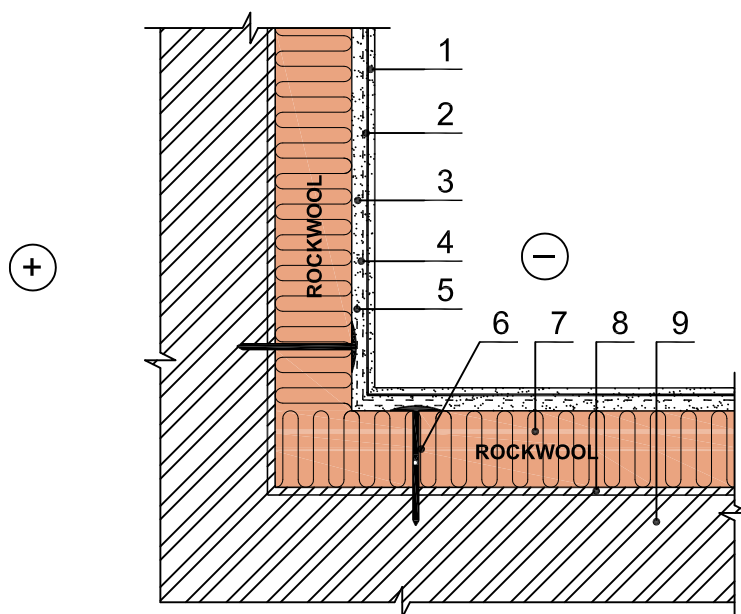
Horizontalus pjūvis
