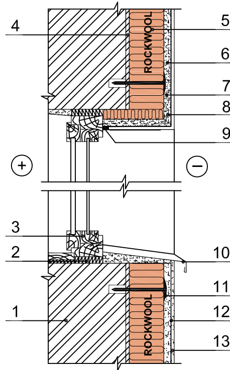
Vertikalus pjūvis
