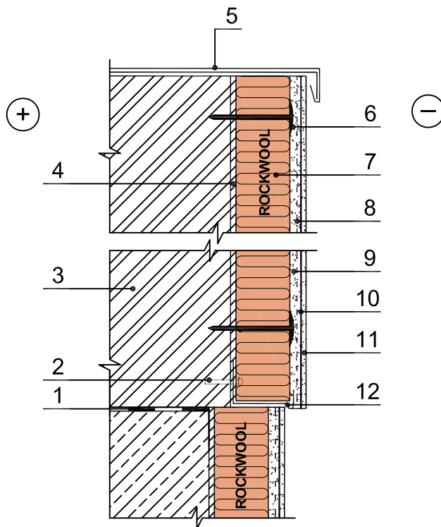
Vertikalus pjūvis
