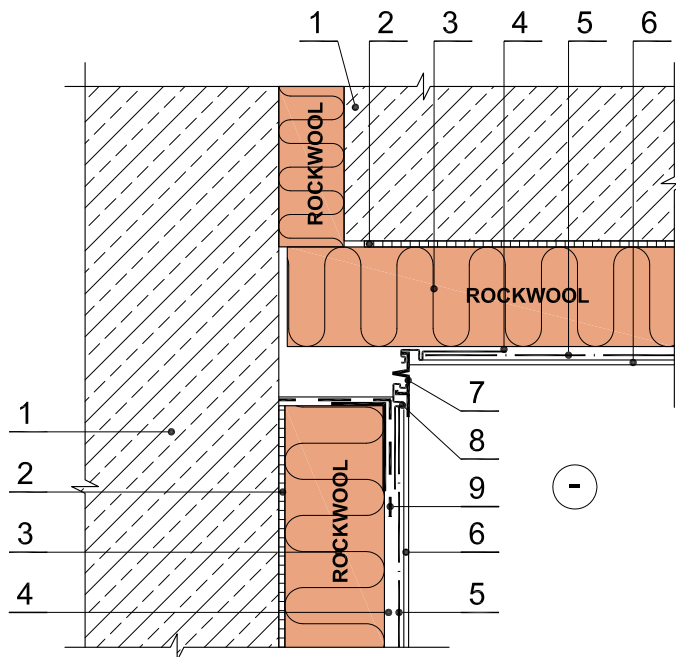
Horizontalus pjūvis
