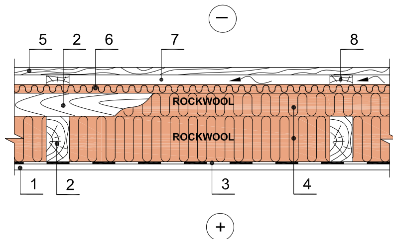
Horizontalus pjūvis
