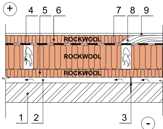
Horizontalus pjūvis
