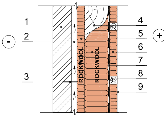
Vertikalus pjūvis
