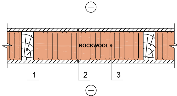
Horizontalus pjūvis
