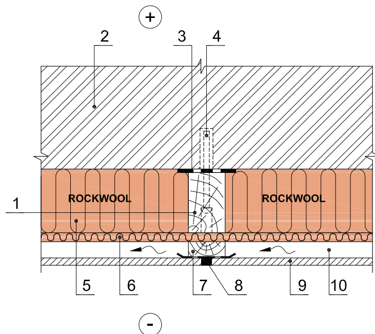
Horizontalus pjūvis
