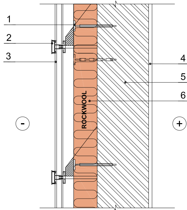
Vertikalus pjūvis
