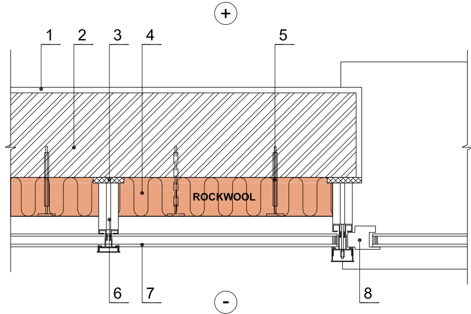
Horizontalus pjūvis
