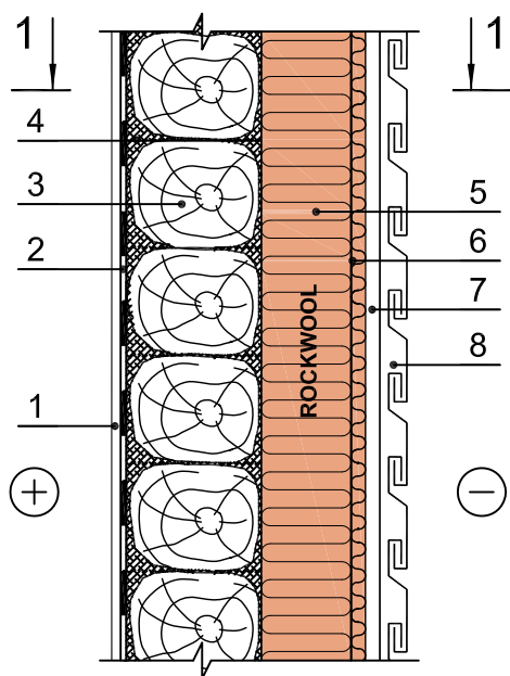
Vertikalus pjūvis
