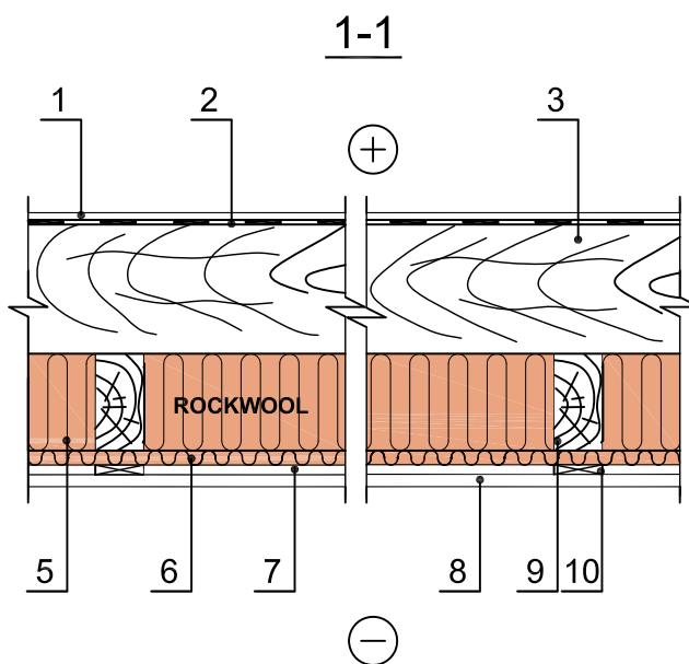
Horizontalus pjūvis
